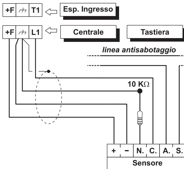
Figura 11 Collegamento di un sensore ad una Zona con Bilanciamento 10K o 10K solo allarme SEOL supervisione.
