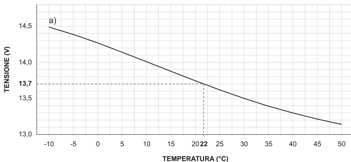
Figura 23 Grafico per regolare la tensione di uscita dell'Alimentatore in funzione della temperatura della Sonda Termica: individuare sull'asse TEMPERATURA (°C) la temperatura della Sonda Termica; tracciare una linea verticale da questo punto fino alla curva a ; tracciare una linea orizzontale dal punto in cui la linea verticale interseca la curva a , all'asse TENSIONE (V) ; Regolare la tensione di uscita dell'Alimentatore sul valore trovato. Per esempio, se la temperatura della Sonda è 22 °C, regolare la tensione di uscita dell'Alimentatore su 13,7 V.
