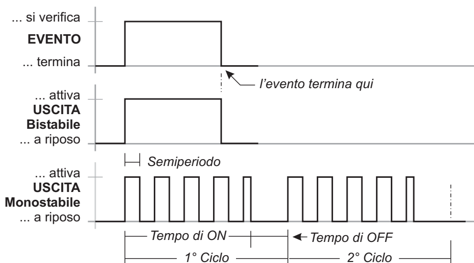
Figura 25 Effetto delle opzioni Semiperiodo e Cicli sulle Uscite Bistabile e Monostabile.
