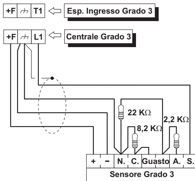
Figura 13 Collegamento di un sensore ad una Zona con Bilanciamento Triplo .
