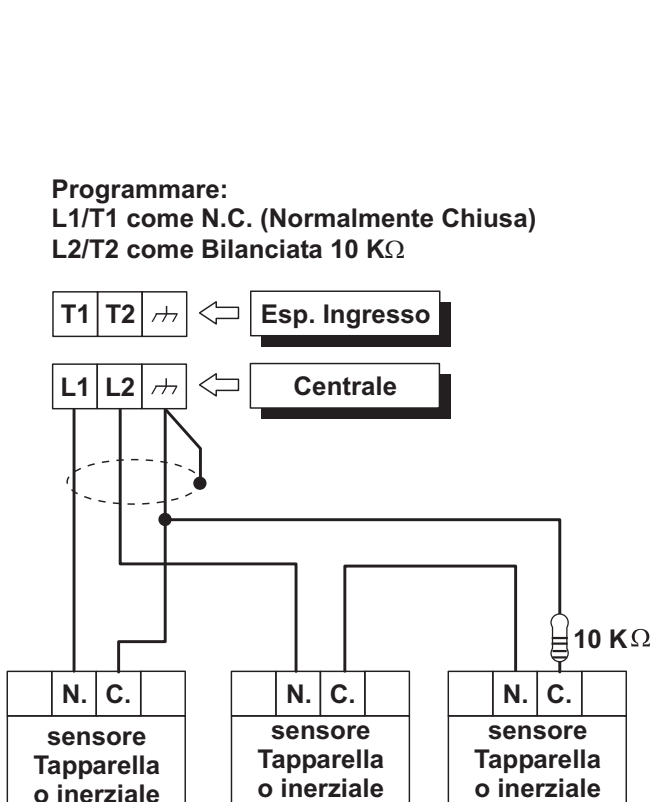
Figura 14 Collegamento di Sensori Inerziali (solo per le zone della Centrale) e Contatti per Tapparella: collegamento di un sensore ad una zona N.C. e di due sensori ad una zona Bilanciata 10K .
