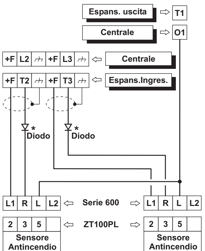
Figura 15 Collegamento di 2 sensori antincendio a Zone con Bilanciamento Normalmente Aperto (* Solo con la serie 600).
